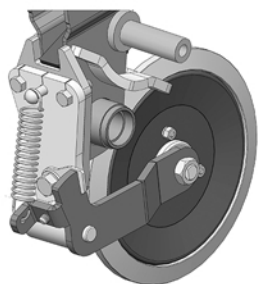
Rueda apretadora 1" x 9 1/2"
